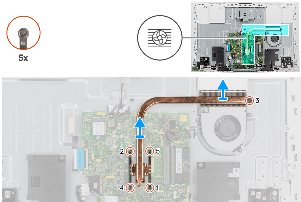
Figure 42. Removing the heat sink- UMA
