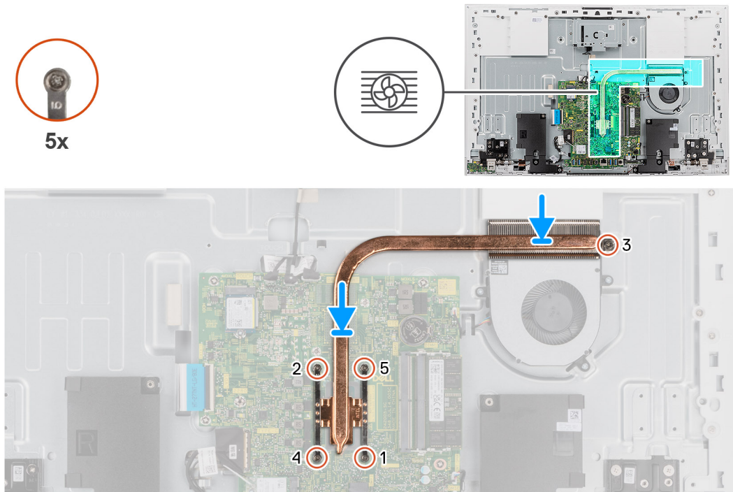
Figure 43. Installing the heat sink- UMA
