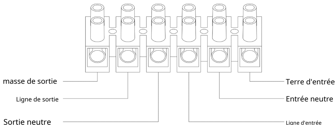
Schéma de câblage du bloc de jonction
