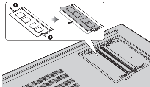
Figura 4-8 Extracción del módulo de memoria
