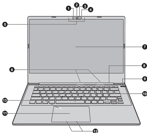
Figura 3-6 Parte frontal del ordenador con el panel de visualización abierto (Serie PORTEGE)
