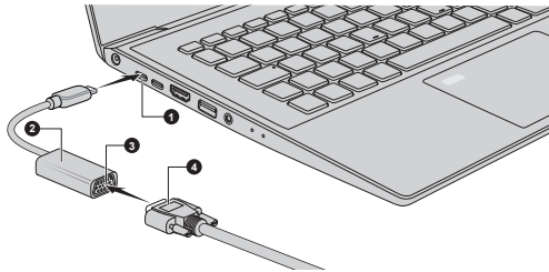
Figura 4-14 Conexión del cable de RGB al puerto para monitor RGB
