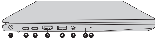
Figura 3-8 Lateral izquierdo del ordenador (Serie TECRA/SATELLITE PRO/dynabook)
