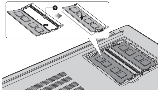
Figura 4-6 Introducción del módulo de memoria
