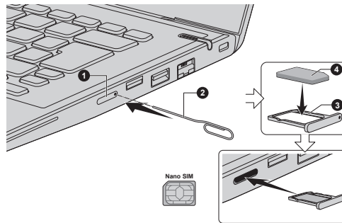
Figura 4-9 Instalación de la tarjeta SIM
