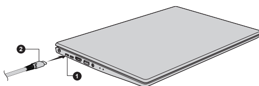
Figura 2-6 Conexión del conector de salida de CC al ordenador
