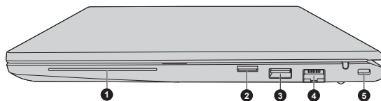
Figura 3-3 Lateral derecho del ordenador (Serie PORTEGE)
