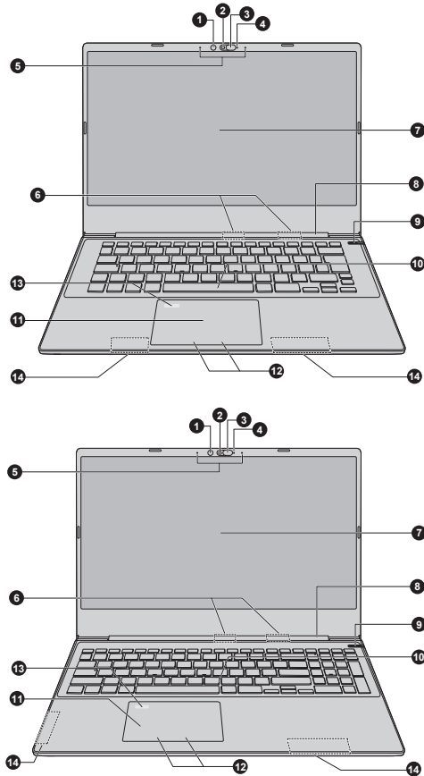
Figura 3-12 Parte frontal del ordenador con el panel de visualización abierto (Serie TECRA/SATELLITE PRO/dynabook)
