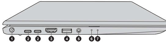
Figura 3-2 Lateral izquierdo del ordenador (Serie PORTEGE)
