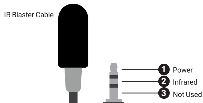
IR BLASTER CABLE PINOUTS
