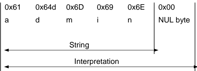
Fig. 8 String example
