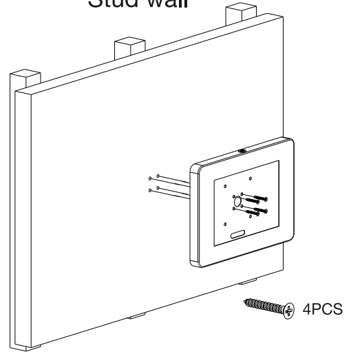
Stud wall
