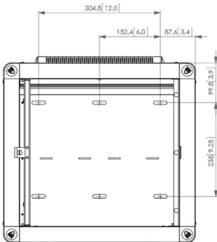
Locatie en afmetingen montagegat (in mm en inches)
