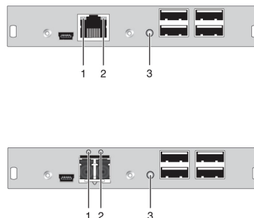
CON module, rear view
