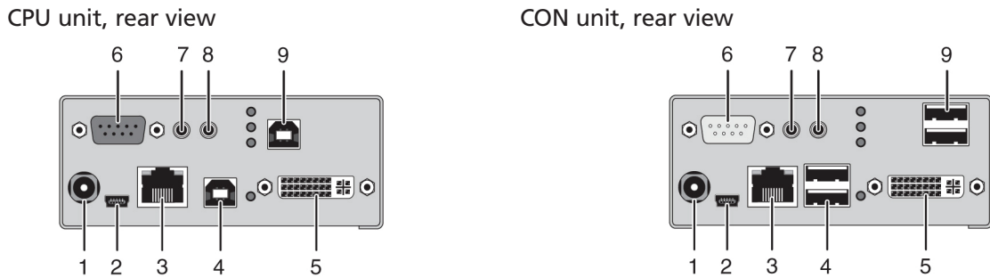
Figure 2-4. ACX1T-12A-C (CPU unit) and ACX1R-12A-C (CON unit).
