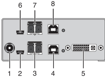
Figure 2-9. ACX1MT-ARH (CPU unit) and ACX1MR-ARH (CON unit).
