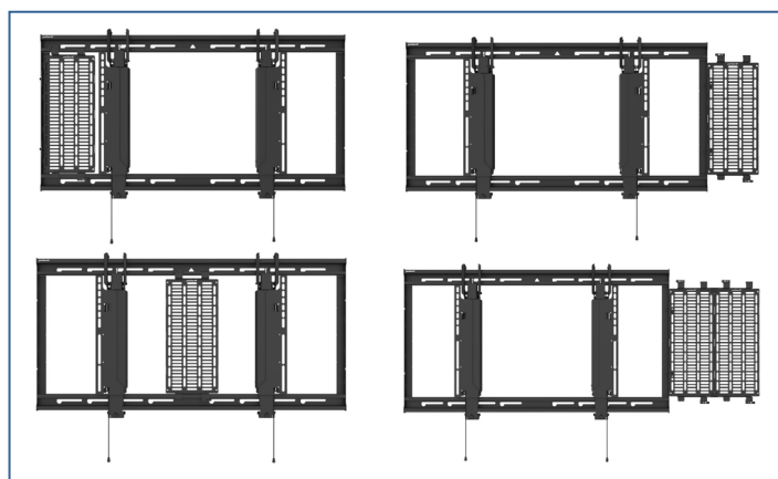
ACC-UCM3 illustré avec le support mural universel à croisillon SmartMount® Ultra-Slim (STS680)
