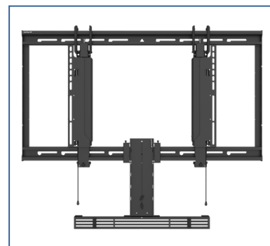
ACC-STSVCB mit der ultradünnen Wandhalterung Universal mit Scherenmechanismus der SmartMount®-Reihe (STS680)
