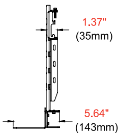
SEITENANSICHT EXTERNE KONFIGURATION
