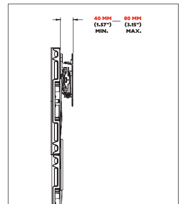
VUE LATÉRALE AVEC PANNEAU DVLED
