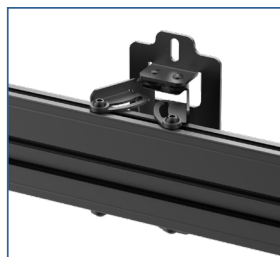
Le mécanisme à engrenages assure un mouvement fluide du bras et un réglage en profondeur sur 40 mm (1,6") sans contraintes
