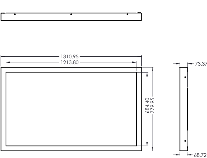
STAND-ALONE XTREME KONFIGURATION - Querformat und Hochformat
