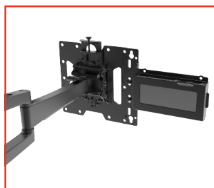
Montage sur les petits supports à mouvement complet
