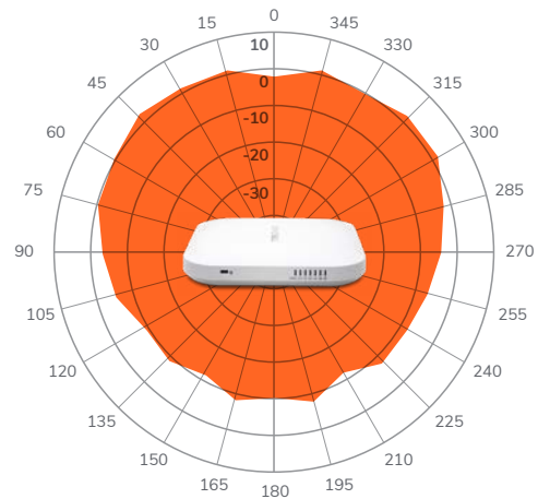
5GHz, YZ-Plane
