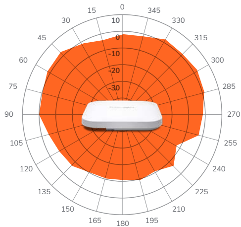
5GHz, XZ-Plane
