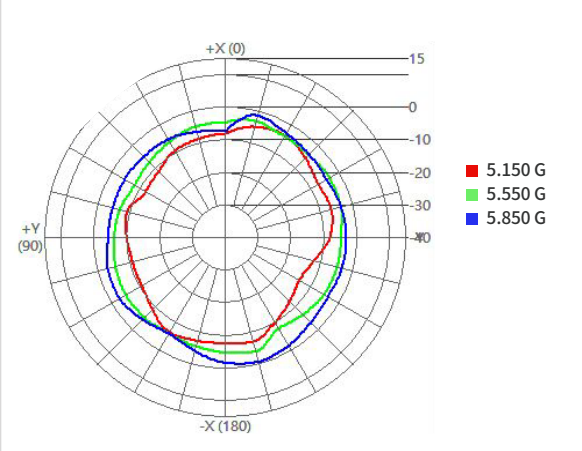
H-Plane
