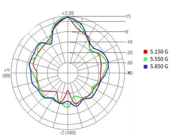
E-Plane
