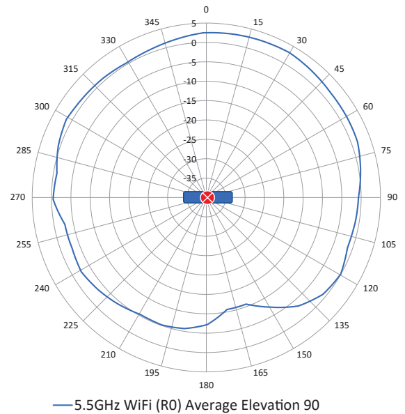
5.5GHz Wi-Fi (antennas 1, 2)
