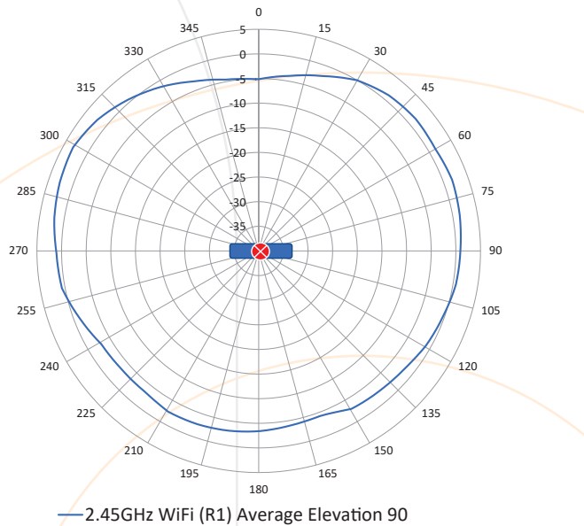
2.45GHz Wi-Fi (antennas 1, 2)
