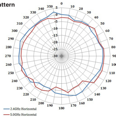
H-Plane Pattern
