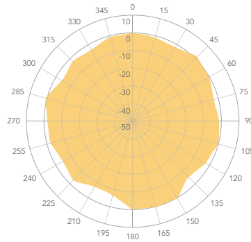
5 GHz Horizontal
