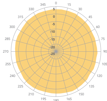
5 GHz Horizontal
