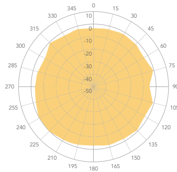
5 GHz Horizontal
