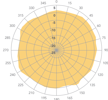
5 GHz Horizontal
