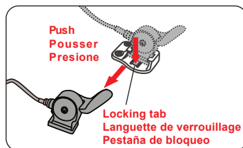
Disassemble the lever Désassembler le levier Desmontaje de la palanca
