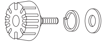
9. Arm Width Adjustment Knob + Washers (2) Bras largeur bouton de réglage + rondelles (2) Perilla de ajuste de ancho del descansabrazos + Arandelas (2)
