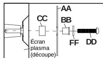
DÉTAIL 1
