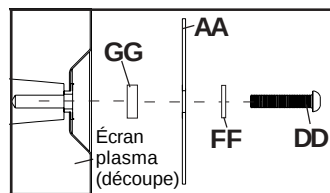
DÉTAIL 2
