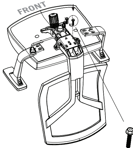
F. Grandes vis 40mm M8 hex
