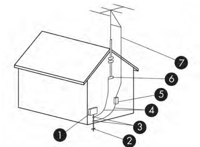
Tabuľka 3-2 Uzemnenie antény
