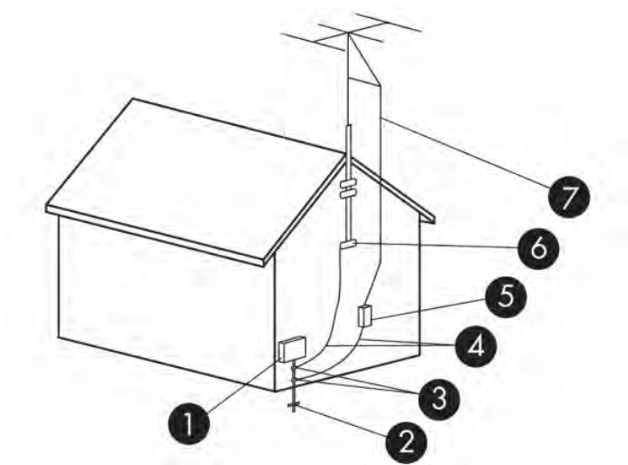
Tablica 3-2 Uzemljenje antene
