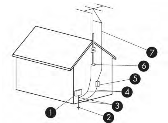
Таблиця 3-2 Заземлення антени
