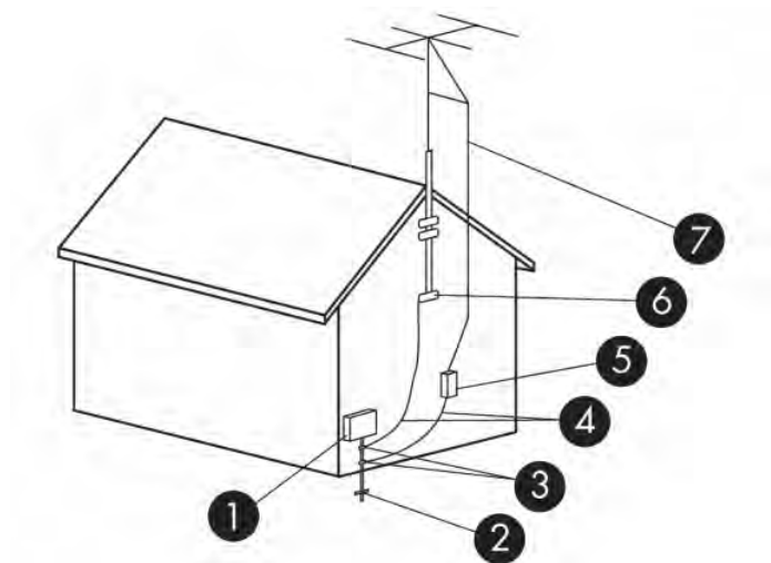
Taulukko 3-2 Antennin maadoitus
