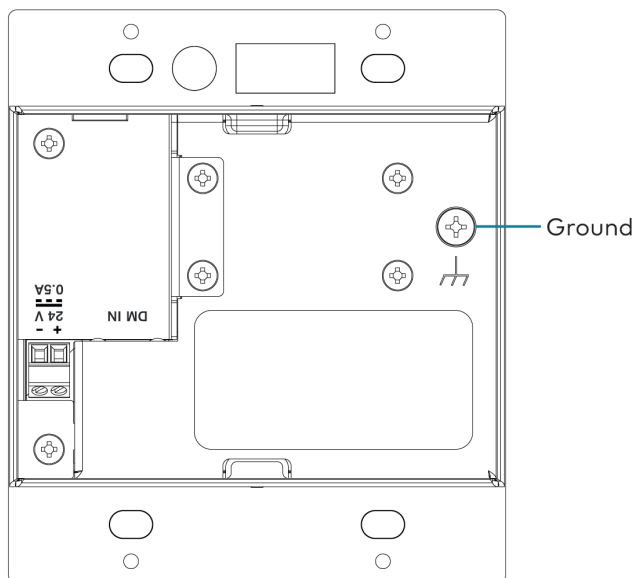
HD-RXU-4KZ-101-2G Rear
