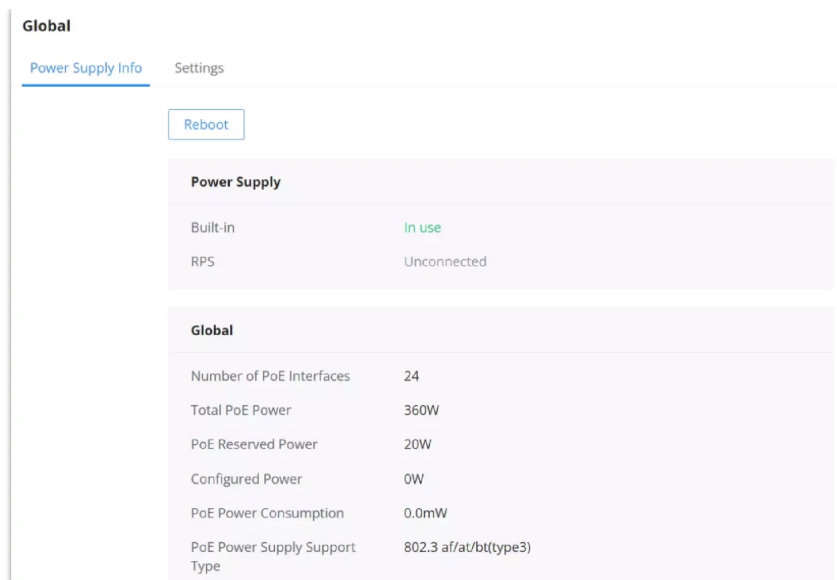
PoE Global
