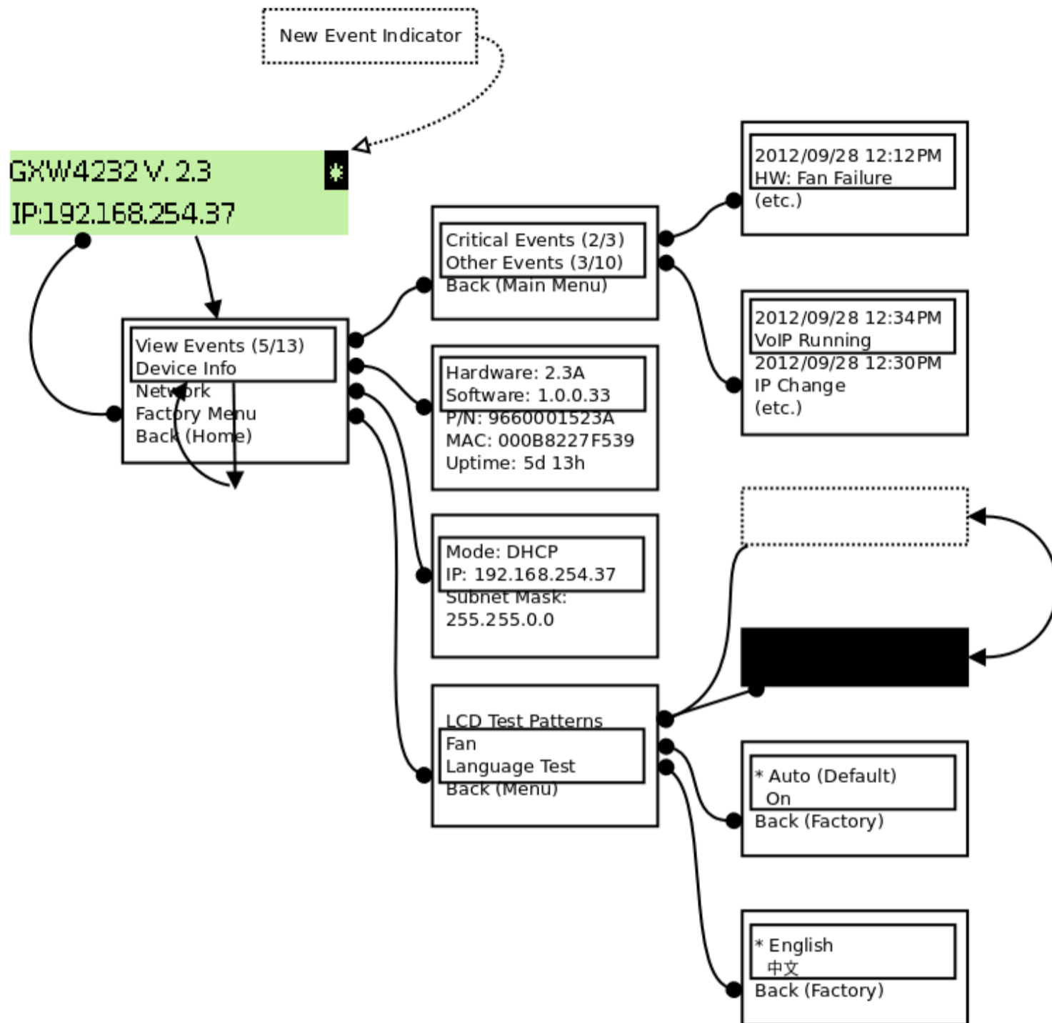
LCD Menu
