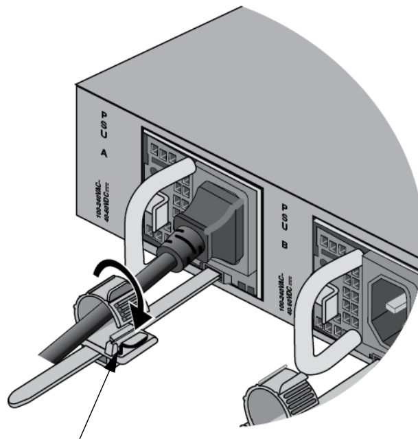
Tab Slot
