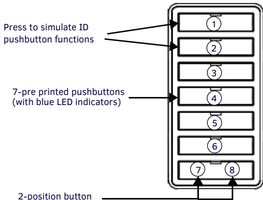
FIG. 3 MET-7E 7-BUTTON KEYPAD
