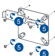
Mini PC 底視圖
