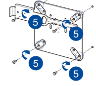
Mini PC 底視圖
