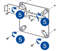
Tampilan bawah Mini PC
