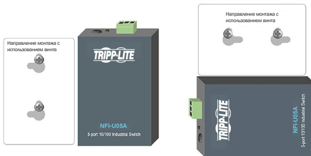
Установка в горизонтальном направлении
