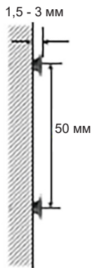
Расстояние между крепежными винтами
