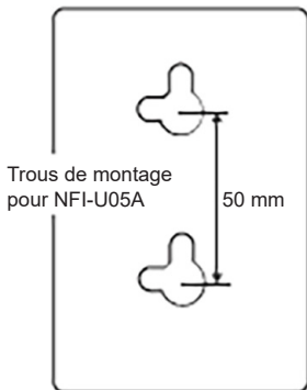
Trous de montage du dessin du NFI-U05A
