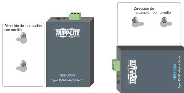
Instalación en Dirección Recta
