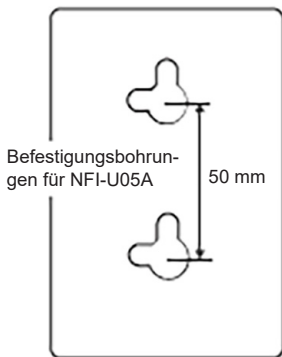
Befestigungsbohrungen für Zeichnung des NFI-U05A
