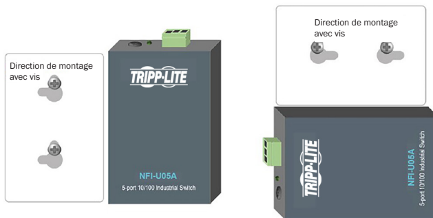
Installation en direction rectiligne
