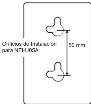
Orificios de Instalación para Dibujo de NFI-U05A
