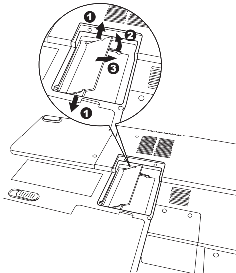
Retrait d'un module mémoire
