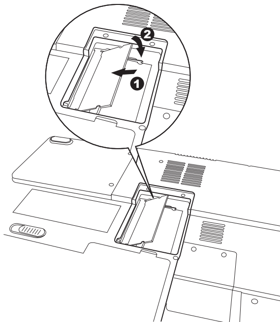
Installation d'un module
