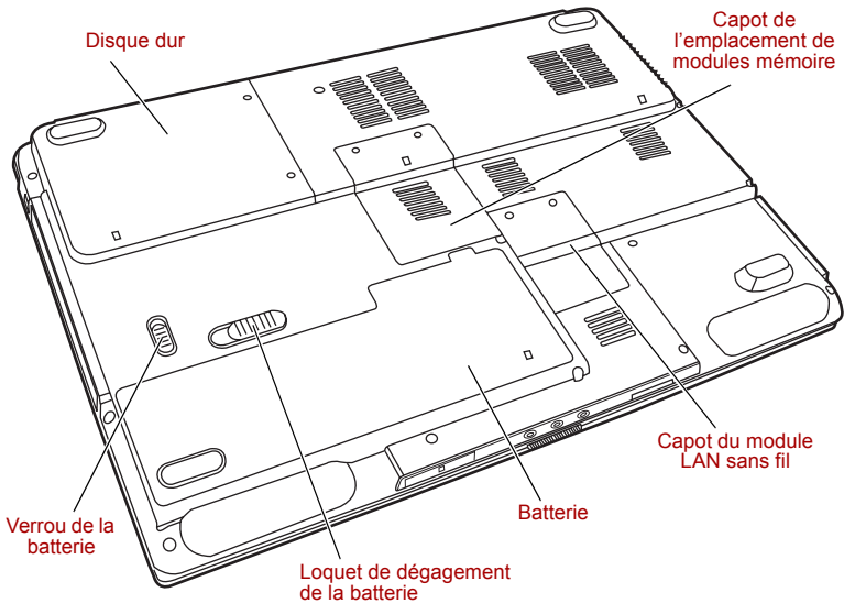
Ordinateur vu de dessous
