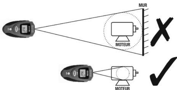
Fig. 4. Mesure de la température d'un moteur à une mauvaise (en haut) et à une bonne (en bas) distance.
