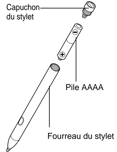
Figure 11. Remplacement de la pile
