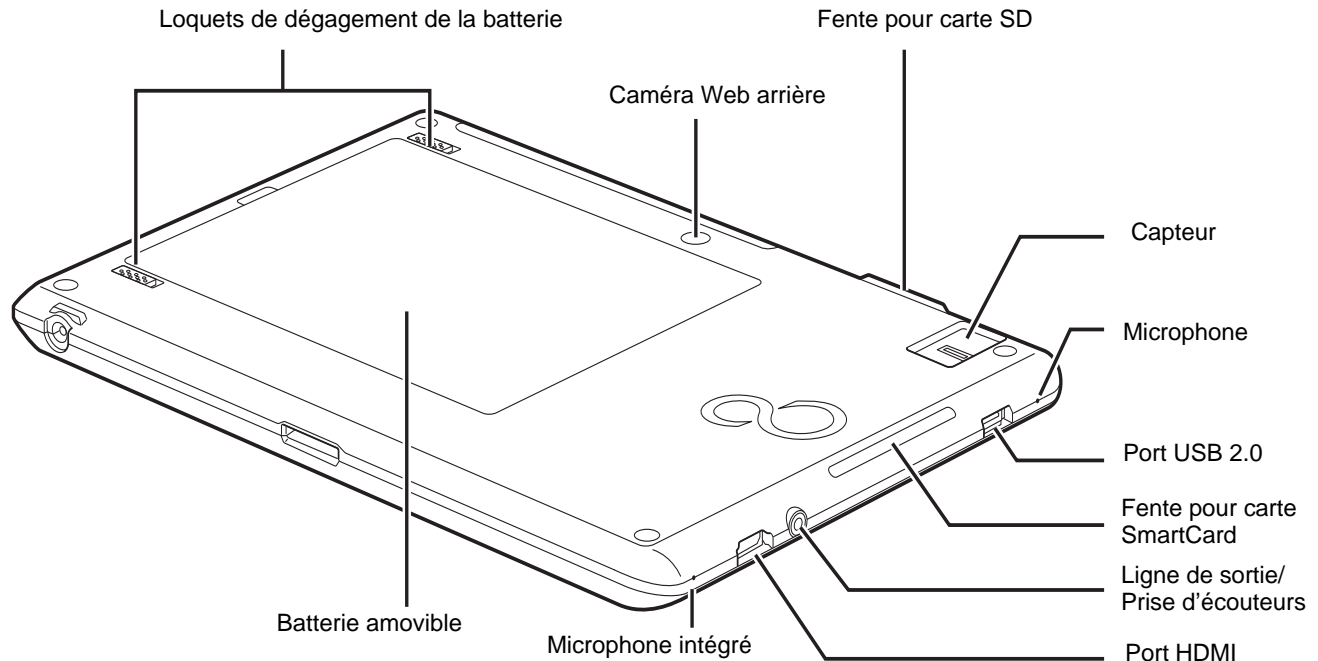
Figure 3. Caractéristiques du PC Tablette STYLISTIC Q550 (vue arrière)
