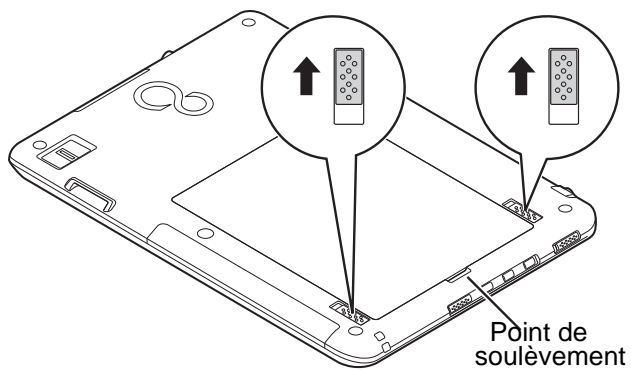
Figure 17. Déverrouillage de la batterie
