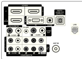
DETALLE DEL PANEL DE TERMINALES 5.2" AL x 6.6" AN
