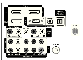
DETALLE DEL PANEL DE TERMINALES 5.2" AI x 6.6" An
