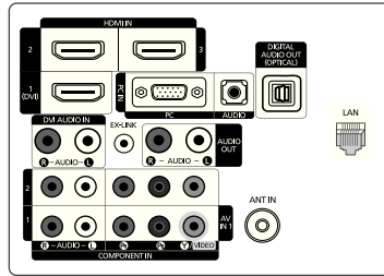
DETALLE DEL PANEL DE TERMINALES 5.2" An x 6.6" An
