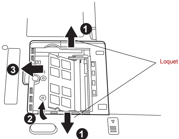
Retrait d'un module mémoire
