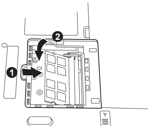
Installation d'un module
