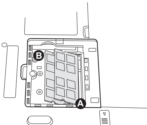
Connecteur A (supérieur), Connecteur B (inférieur)
