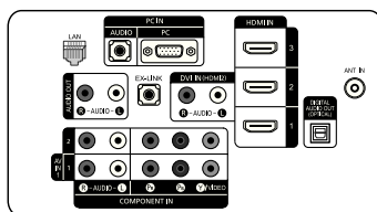
DETAILS DU PANNEAU DES PRISES 3.7" H X 9.1" W
