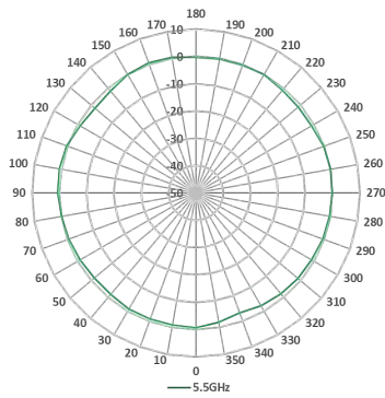
5.5GHz Horizontal
