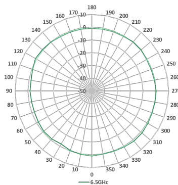
6.5GHz Horizontal
