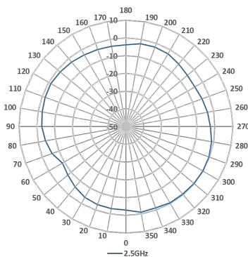
BLE Horizontal
