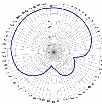
2.4 GHz E-plane
