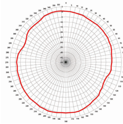
5 GHz H-plane
