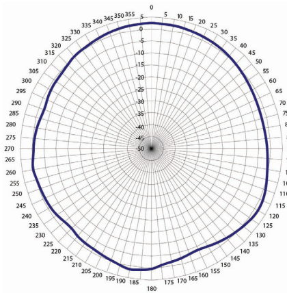
2.4 GHz H-plane
