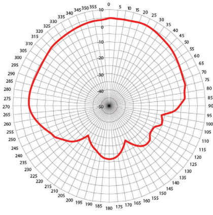
5 GHz E-plane
