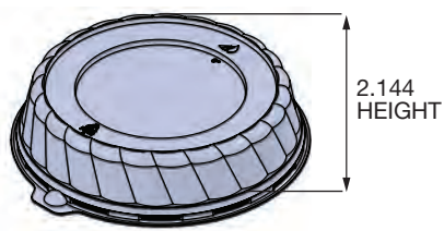
9" Dome Lid 89036
